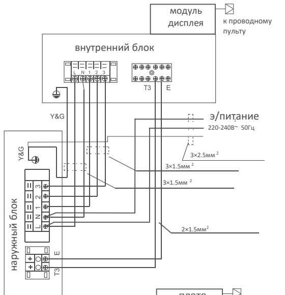
Блок MDTJ2-24HWN1
