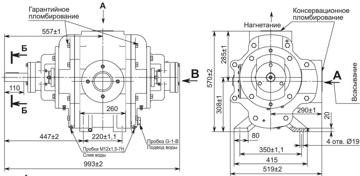
Насос ВВН1-12
