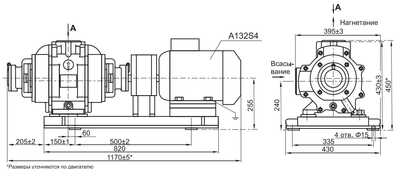
Агрегат ВВН1-3
