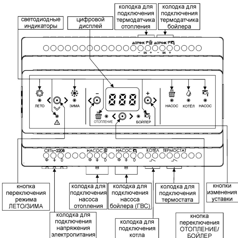
Рисунок 1 — Общий вид передней панели изделия
