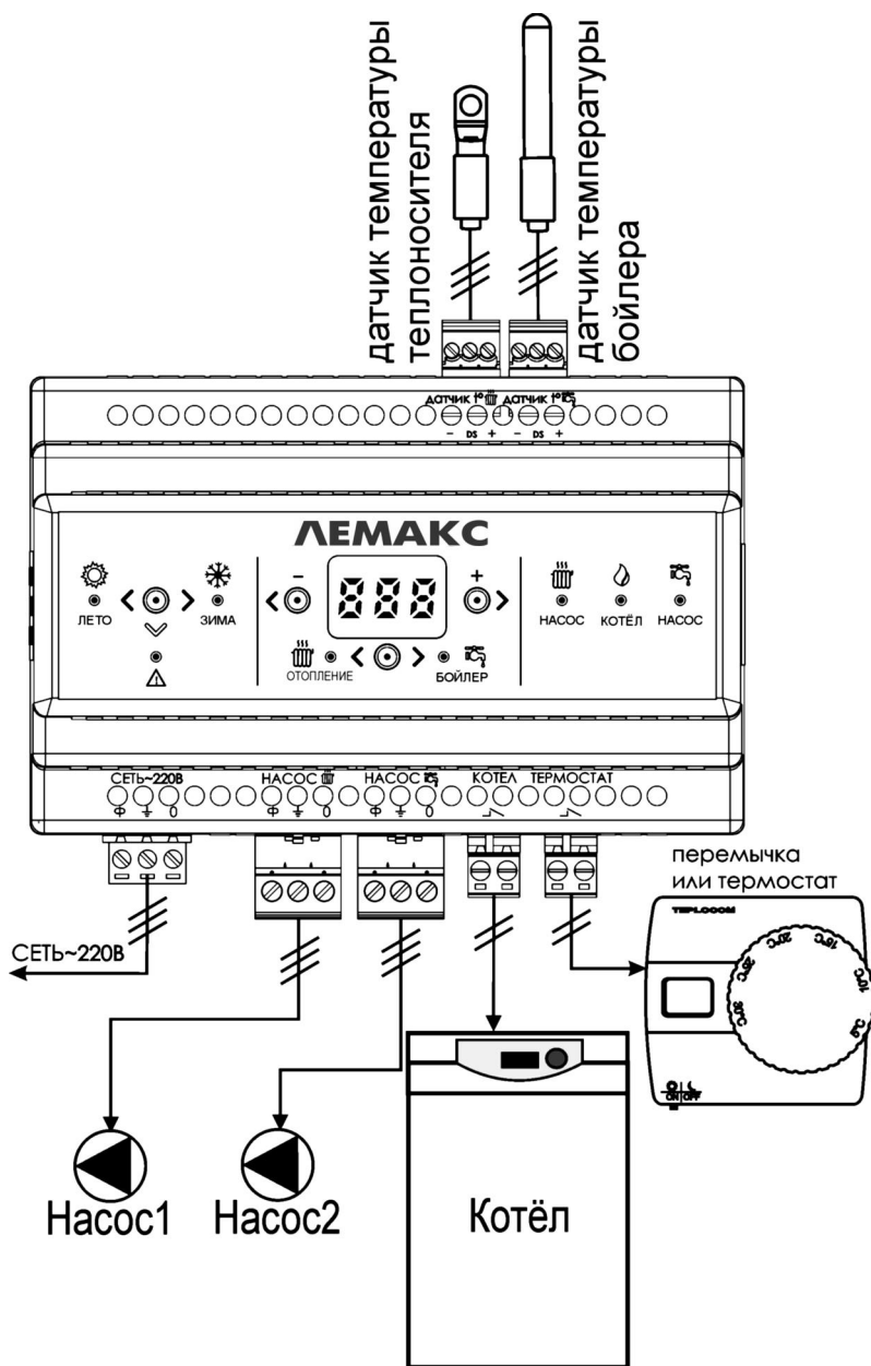
Рисунок 4 - Схема подключения
