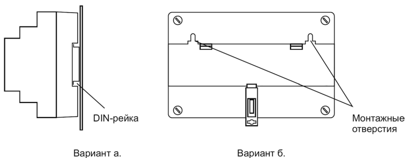
Рисунок 3 — Варианты установки изделия
