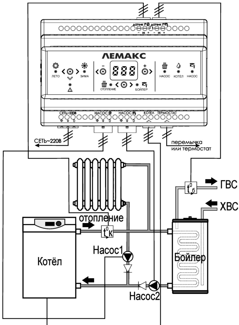
Рисунок 2 – Функциональная схема системы отопления
