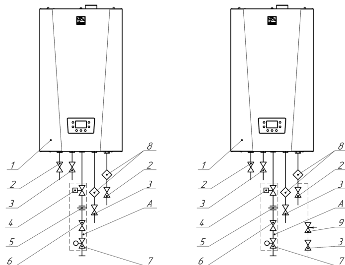
Рис. 7. Требования к подключению котла
