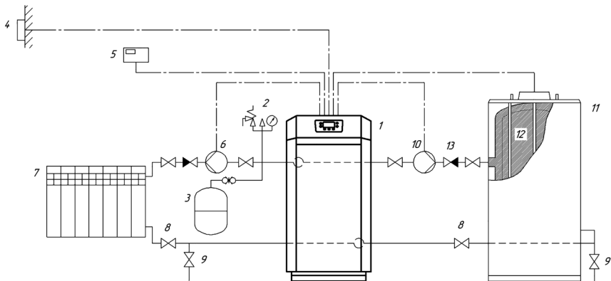
Рис. 7. Примерная гидравлическая схема подключения котла к системе отопления и бойлеру косвенного нагрева с двумя насосами*
