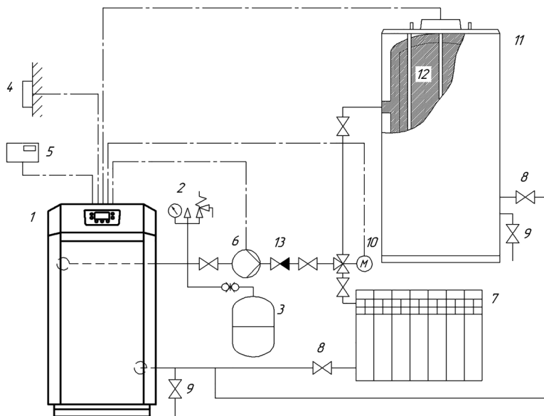
Рис. 8. Примерная гидравлическая схема подключения котла к системе отопления и бойлеру косвенного нагрева с разделительным клапаном*
