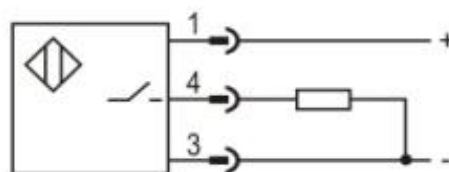
PNP NO
