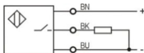
PNP NO
