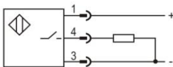
PNP NO
