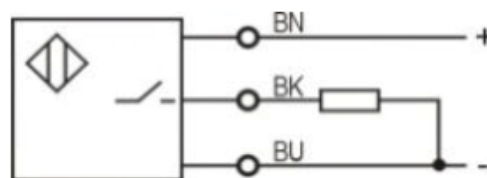
PNP NO
