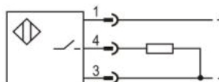
PNP NO
