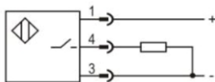
PNP NO
