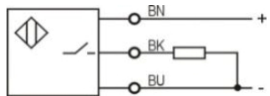
PNP NO
