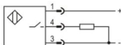
PNP NO
