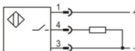
PNP NO
