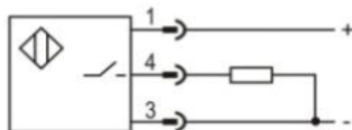
PNP NO
