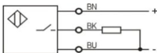
PNP NO
