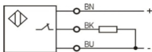
PNP NO
