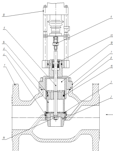
Рисунок 3. Разгруженный по давлению клапан DN 50 – 400. Исполнение Б.
