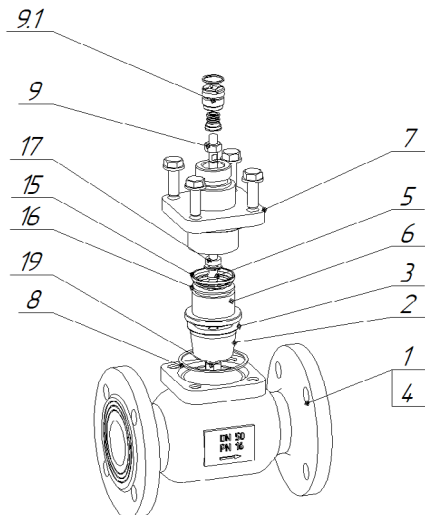
Рисунок 3. Разгруженный по давлению клапан DN 50 – 400. Исполнение Б.
