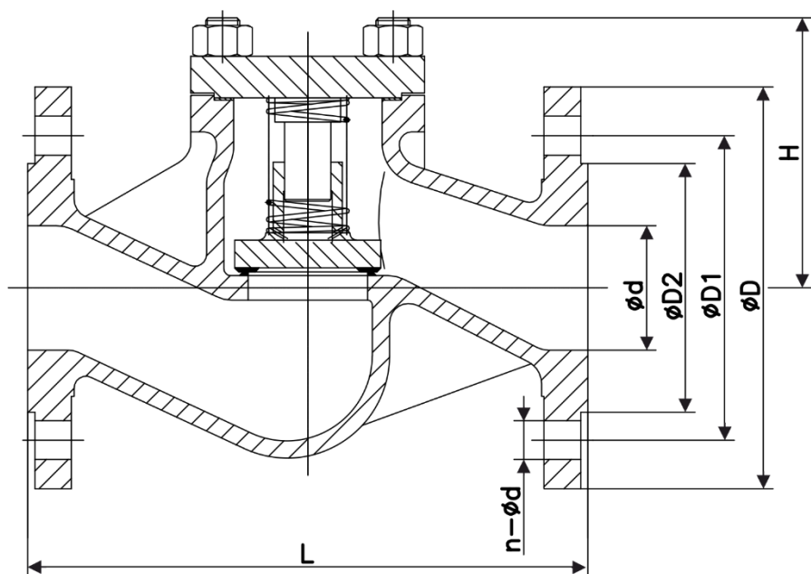
Рисунок 3 – Размеры
