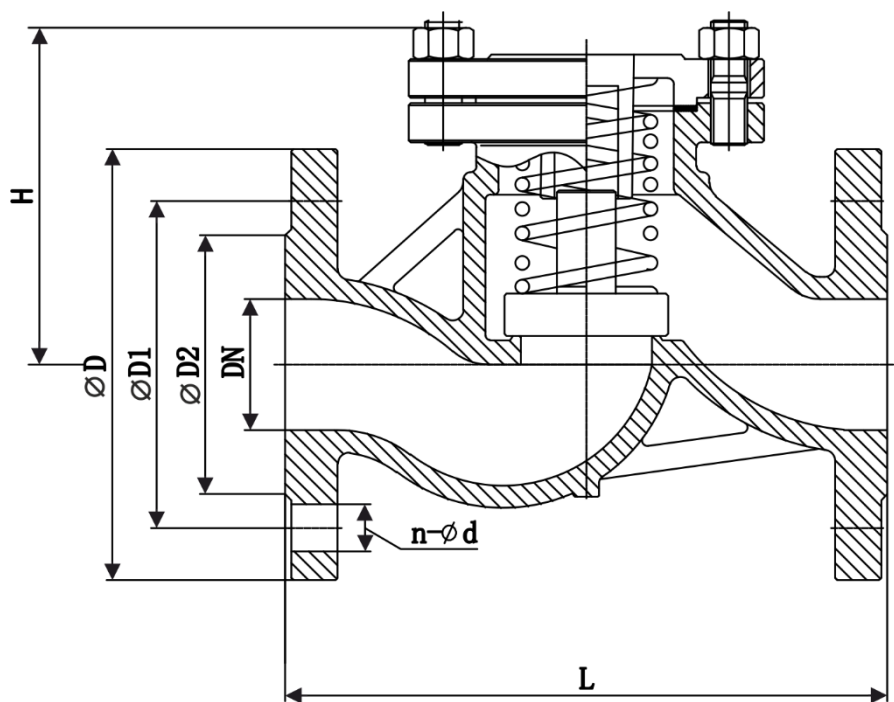
Рисунок 3 – Размеры
