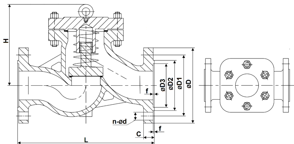
Рисунок 3 – Размеры
