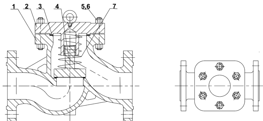
Рисунок 2 – Деталировка
