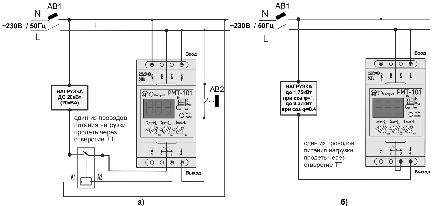
Рисунок 2 – Схема подключения OptiDin PMT-101
