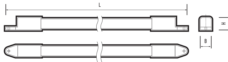
Рис. 1 Светильник PLED T4i
