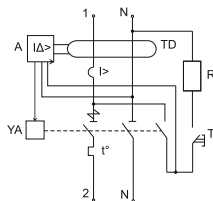
Рисунок А.2 – Схема электрическая принципиальная АВДТ тип АС/ Figure A.1 – Electric schematic diagram of AVDT of AC type
