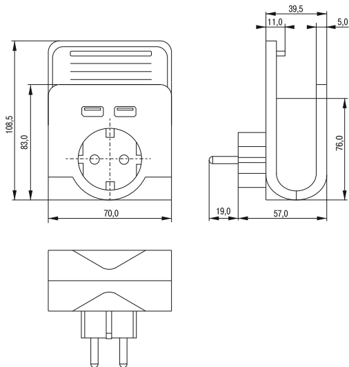
Рисунок 1 – Адаптер типа T-02/01
