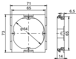
Рисунок 15 – Суппорт для ЭУИ для кабель-канала 100x40 и 100x60 / Figure 15 – Support for modular wiring accessories for cable trunking 100x40, 100x60 / 15 – сурет – 100x40 және 100x60 кабельдік арнаға арналған модульді ЭУИ-лерді үшін суппорт
