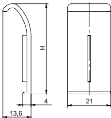
Рисунок 9 – Соединитель на стык боковой / Figure 9 – Lateral joint connector / 9 – сурет – Бүйірлік қосылым
