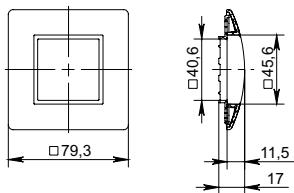
Рисунок 2 – Рамка и суппорт для КМКУ на 2 модуля / Figure 2 – Frame and support for KMKU (2 modules) / 2 – сурет – КМКУ үшін жақтау және қолдау (2 модуль)
