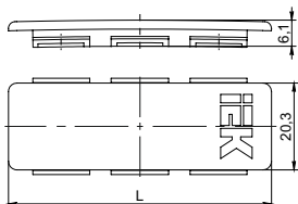
Рисунок 6 – Заглушка 150x60 / Figure 6 – End cap 150x60 / 6 – сурет – Бітеуіш 150x60
