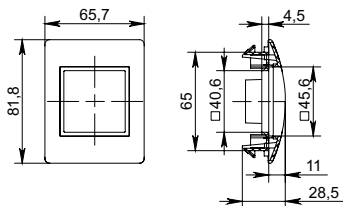
Рисунок 1 – Рамка и суппорт универсальные на 2 модуля / Figure 1 – Universal frame and support (2 modules) / 1 – сурет – Өмбебап жақтау және қолдау (2 модуль)
