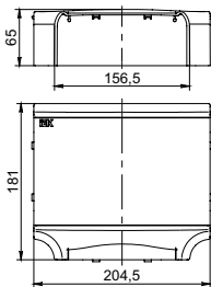
Рисунок 12 – Угол Т-образный 150x60 / Figure 12 – T-type angle 150x60 / 12 – сурет – Т-тәріздес бұрма 150x60
