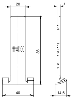
Рисунок 16 – Фиксатор кабеля / Figure 16 – Cable retainer / 16 – сурет – Кабельді бекіткіш
