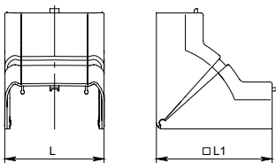
Рисунок 13 – Угол внешний изменяемый / Figure 13 – Variable external angle / 13 – сурет – Сыртқы бұрыш айнымалысы
