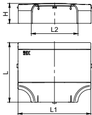
Рисунок 11 – Угол Т-образный / Figure 11 – T-type angle / 11 – сурет – Т-тәріздес бұрма
