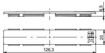
Рисунок 8 – Соединитель на стык лицевой для крышки 125мм / Figure 8 – Front joint connector for cover 125mm / 8 – сурет – Қақпаққа арналған алдыңғы қосылым 125мм
