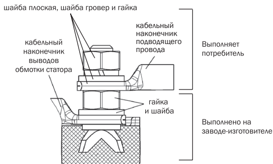
Рисунок 5 – Схема контактного соединения
