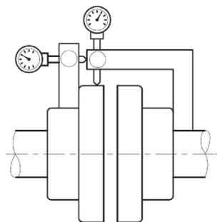
Рисунок 8 – Схема комбинированного измерения аксиальной и радиальной несоосности
