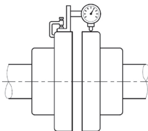
Рисунок 7 – Схема измерения радиальной несоосности (смещения осей)
