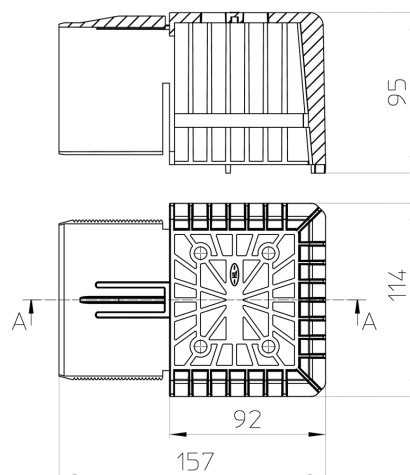
Schnitt A-A
