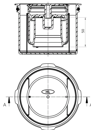
Schnitt A-A
