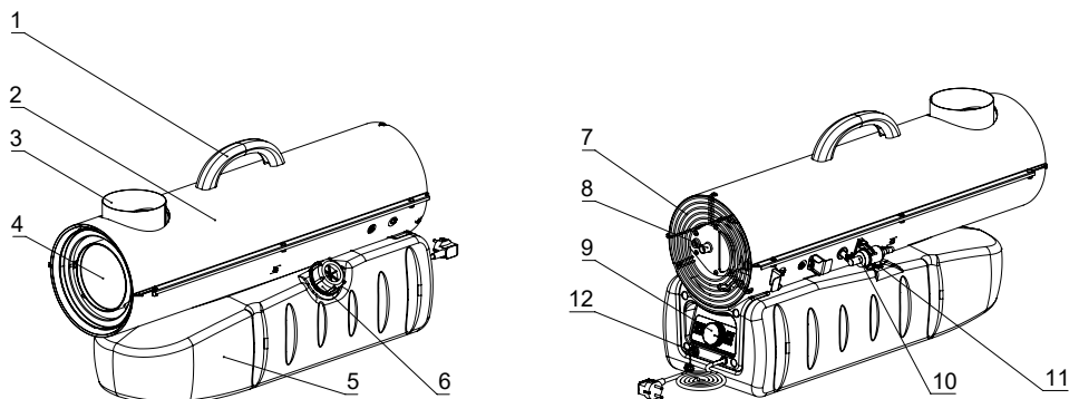
Рисунок 1 – Устройство модели KHDN–20
