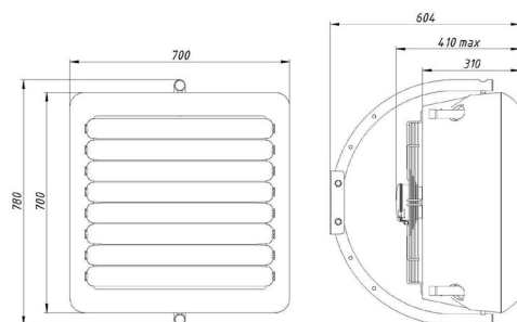
Рисунок 1. Отопительный агрегат T-Heat AC
