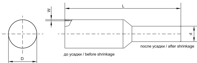
Рисунок 1 – Габаритные размеры ТТУ / Figure 1 – Overall dimensions of TTU
