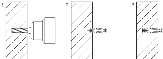
Рисунок 3 – Порядок монтажа хомута
