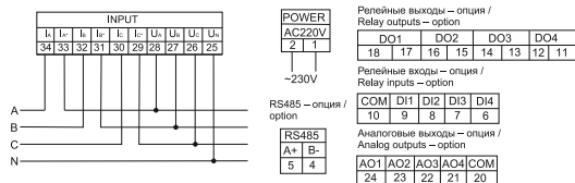
а) схема подключения мультиметра LED к четырехпроводной сети при I \leq 5 А, U \leq 600 В / LED multimeter connection diagram to a four-wire network at I \leq 5 A, U \leq 600 V
