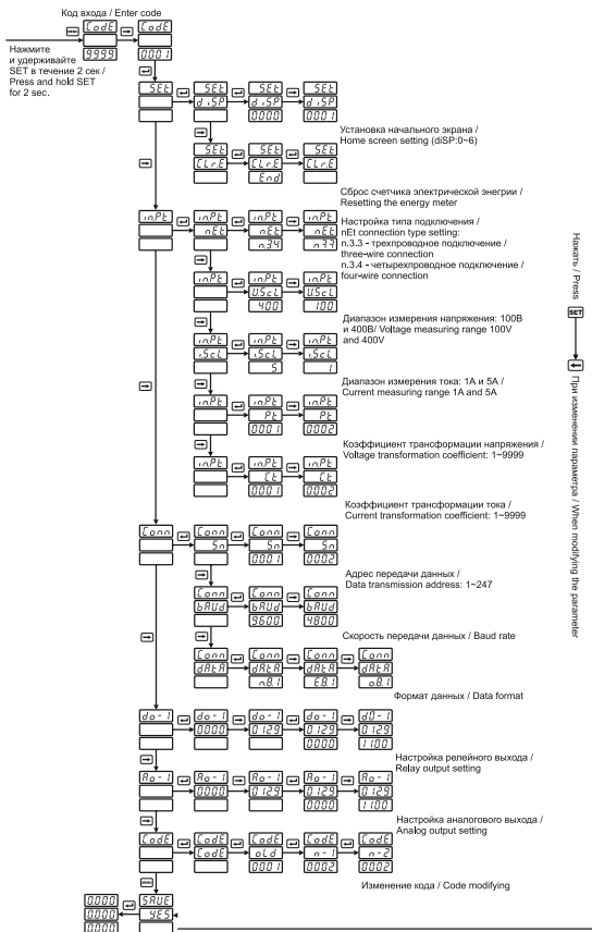
Рисунок 4 – Меню прибора / Figure 4 – Instrument menu
