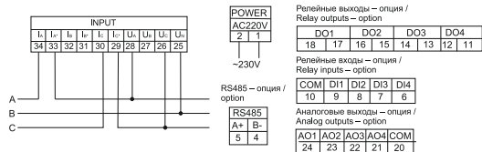
б) схема подключения мультиметра LED к трехпроводной сети при I \leq 5 А, U \leq 600 В / LED multimeter connection diagram to a three-wire network at I \leq 5 A, U \leq 600 V
