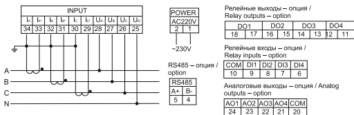
с) схема подключения мультиметра LED к четырехпроводной сети при I > 5 \text{ A} , U \leq 600 \text{ B} / LED multimeter connection diagram to a four-wire network at I > 5 \text{ A} , U \leq 600 \text{ V}
