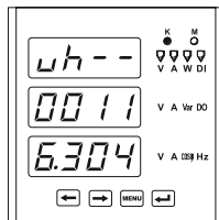
e) diSP 5. Отображение активной энергии / diSP 5. Active energy display
