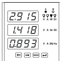
c) diSP 3. Отображение активной мощности, реактивной мощности, \cos\varphi / diSP 3. Display of active power, reactive power, \cos\varphi
