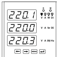
a) diSP 1. Отображение напряжения на фазе A, B, C / diSP 1. Voltage display at phase A, B, C
