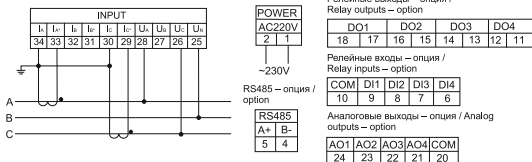
д) схема подключения мультиметра LED к трехпроводной сети при I > 5 \text{ A} , U \leq 600 \text{ B} / LED multimeter connection diagram to a three-wire network at I > 5 \text{ A} , U \leq 600 \text{ V}
