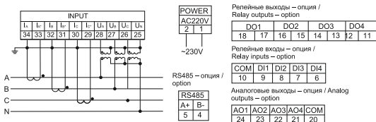
е) схема подключения мультиметра LED к четырехпроводной сети при I > 5 \text{ A} , U > 600 \text{ B} / LED multimeter connection diagram to a four-wire network at I > 5 \text{ A} , U > 600 \text{ V}
