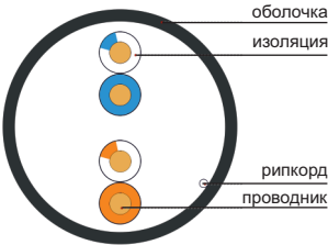
Рисунок 2.2.1 – Конструкция кабеля BC1-C5E02-111-UUU-G
