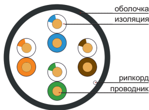
Рисунок 2.5.1 – Конструкция кабеля BC1-C5E04-111-UUU-G
