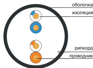
Рисунок 2.10.1 – Конструкция кабеля BC3-C5E02-339-500-G
