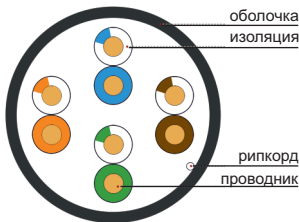
Рисунок 2.11.1 – Конструкция кабеля BC3-C5E04-139-UUU-G
