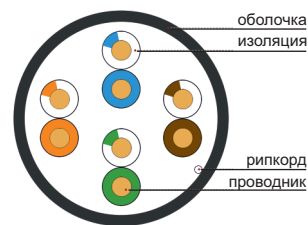
Рисунок 2.6.1 – Конструкция кабеля BCC1-C5E04-111-305-G
