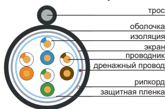
Рисунок 2.13.1 – Конструкция кабеля BC3-C5E04-359-305-G
