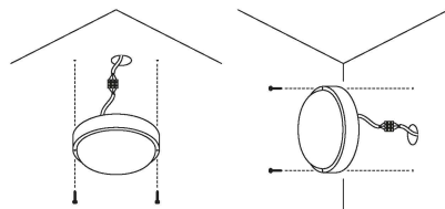
Рис. 2. Пример монтажа
