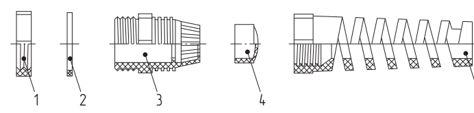
1 – Гайка крепежная (S) 2 – Кольцо уплотнительное 3 – Корпус кабельного ввода 4 – Уплотнитель кабеля 5 – Гайка накладная-ввод спиральный (S)
