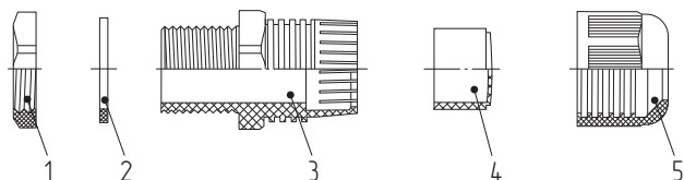
1 – Гайка крепежная (S) 2 – Кольцо уплотнительное 3 – Корпус кабельного ввода 4 – Уплотнитель кабеля 5 – Гайка накладная (S)
