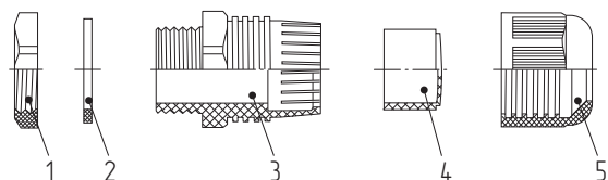
1 – Гайка крепежная (S) 2 – Кольцо уплотнительное 3 – Корпус кабельного ввода 4 – Уплотнитель кабеля 5 – Гайка накладная (S)
