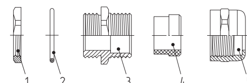
1 – Гайка плоская прижимная (S 1 ) 2 – Кольцо уплотнительное 3 – Корпус кабельного ввода 4 – Уплотнитель кабеля 5 – Гайка накидная (S)
