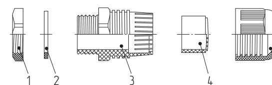
1 – Гайка крепежная (S 1 ) 3 – Корпус кабельного ввода 5 – Гайка накладная (S) 2 – Кольцо уплотнительное 4 – Уплотнитель кабеля
