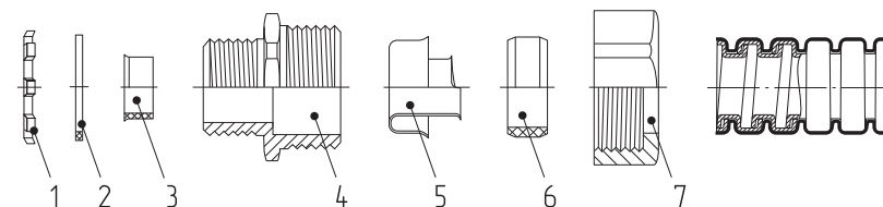
1 – Гайка заземляющая 3 – Втулка защитная 4 – Корпус 6 – Уплотнитель металлокава 2 – Кольцо уплотнительное 5 – Оконцеватель металлокава 7 – Гайка накидная
