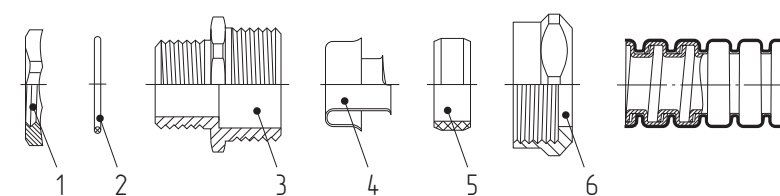
1 – Гайка заземляющая 3 – Корпус 5 – Уплотнитель металлокабеля 2 – Кольцо уплотнительное 4 – Оконцеватель металлокабеля 6 – Гайка накидная
