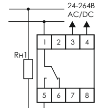
Схема подключения изделия и нагрузки, питающихся от разных источников.
