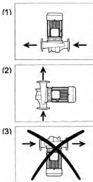
(1) Вариант монтажа насоса в горизонтальном положении
