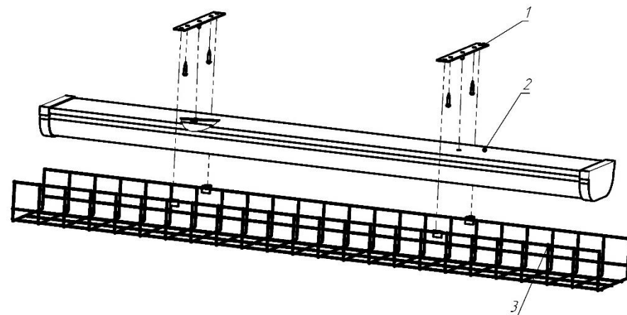
Рисунок 1. Схема монтажа защитной решётки
