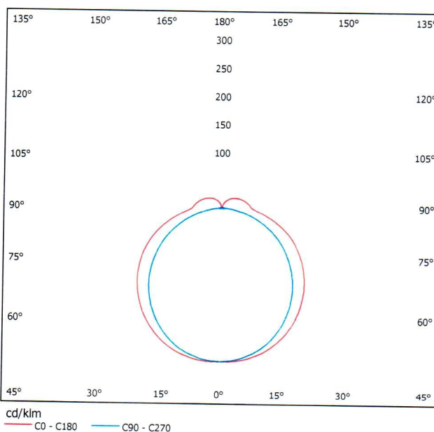
Рисунок 2 – График КСС образца в полярных координатах
