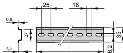
Рисунок 2. Монтажно-габаритные размеры DIN-рейки DR-p
