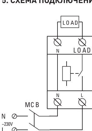
Рисунок 8 – Условная схема подключения
