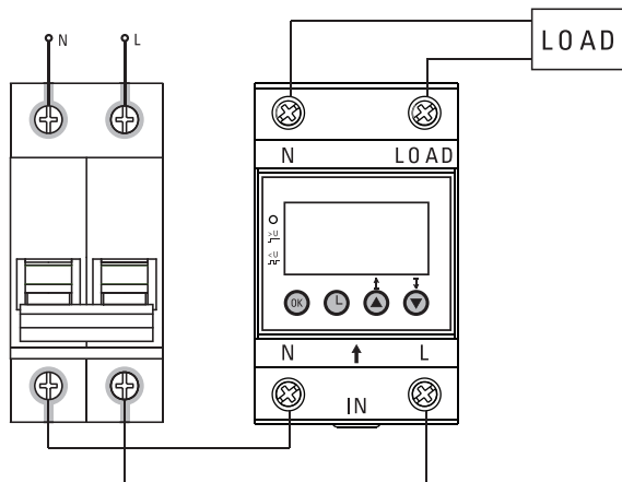
Рисунок 9 – Схема подключения
