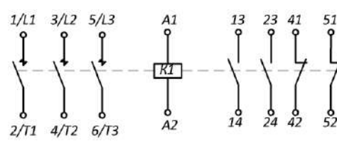
Рис. 4. Принципиальная схема 3-х полюсных контакторов с 2з+2р доп.контактами
