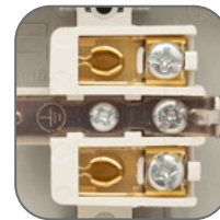
Пластиновые пружины в контактной группе
