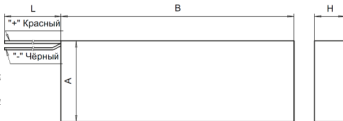
Рис.8 BS-10HRHT26/50-4.0/F-НВ500-VHR-3N-1
