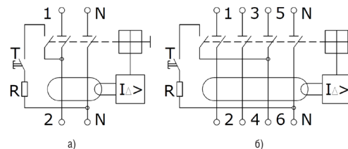
а) двухполюсного; б) четырехполюсного. Т – устройство эксплуатационного контроля (кнопка «Т» - тест). R – токоограничивающее сопротивление. Рисунок В.1 - Принципиальные электрические схемы ВДТ
