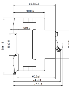
а) двухполюсного; б) четырехполюсного. Рисунок Б.1 - Габаритные, установочные и присоединительные размеры ВДТ
