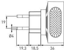
Рис. 2 - Габаритные размеры
