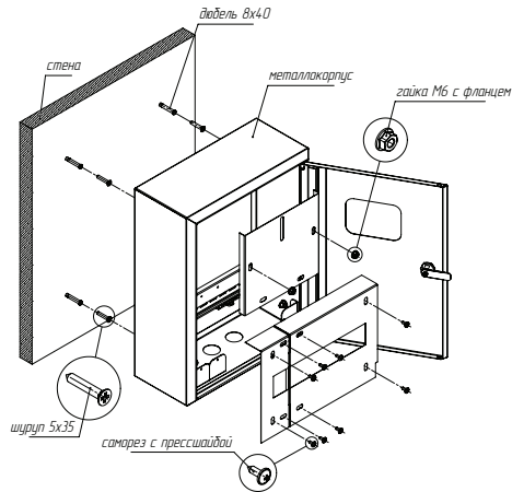
Рис. 1 - Схема монтажа
