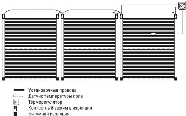
Рисунок 1. Общая схема подключения, в случаях, когда установочные провода проложены под плитусом, утоплены в прорезях теплоизоляции, или в специальных кабель-каналах, исключающих непосредственное механическое воздействие.
